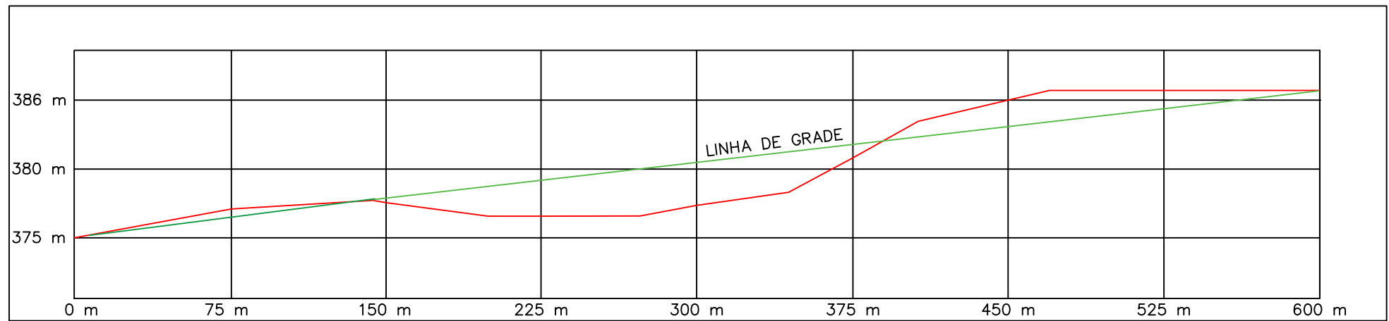
PERFIL DE ELEVAÇÃO
